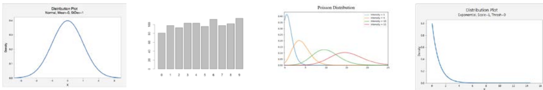
การแจกแจงแบบปกติ
