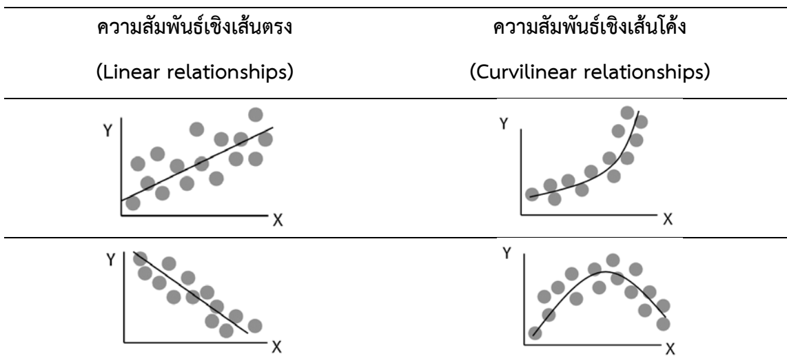
รูปที่ 9.4 ความสัมพันธ์เชิงเส้นตรงและเส้นโค้ง
