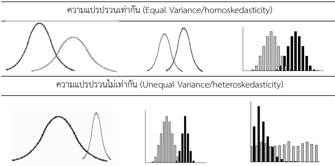
รูปที่ 9.3 ความแปรปรวน
