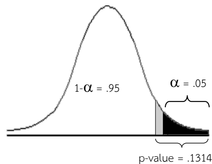
รูปที่ 3.3 ค่าวิกฤติการทดสอบแบบหางเดียวทางขวา
