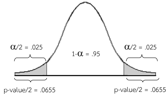
รูปที่ 3.5 ค่าวิกฤติการทดสอบแบบ 2 ทาง
