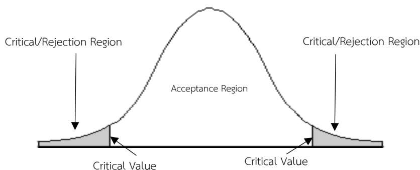
รูปที่ 3.2 เขตวิกฤต
